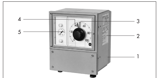
Bild 1 · Festwertregler für Temperatur mit Reglerstation Typ 3432-01
