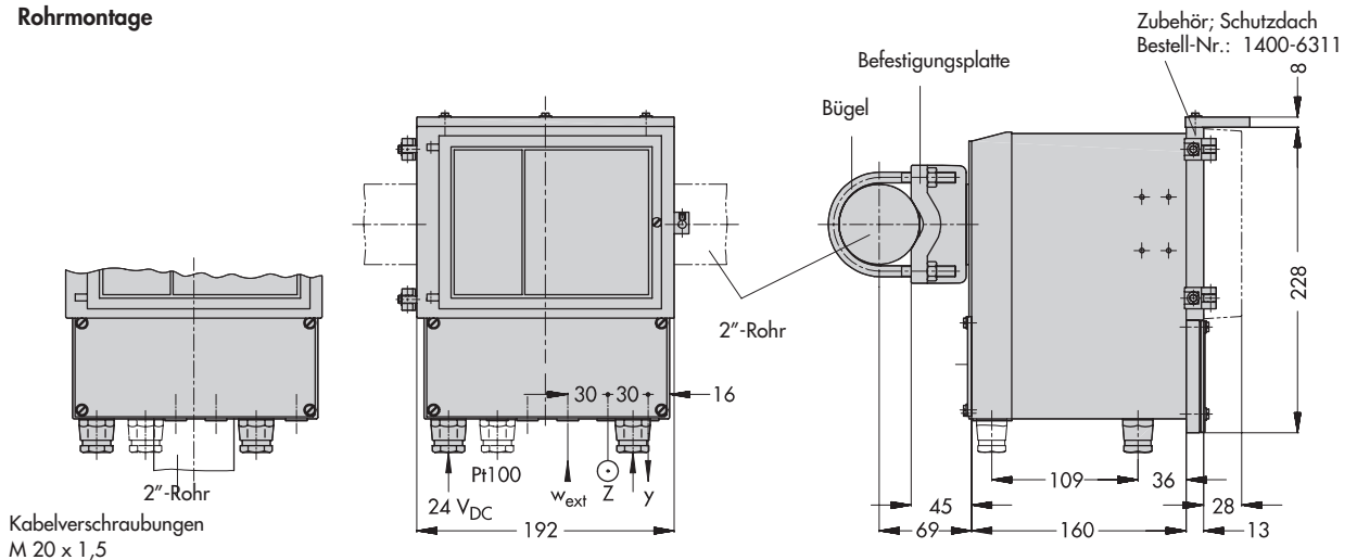
Bild 5 · Abmessungen – Rohrmontage –
